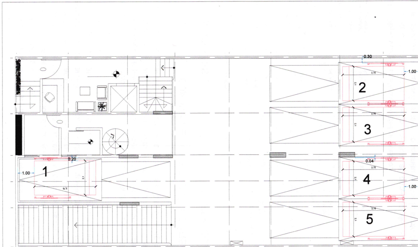
PLANTA DE SEMISOTANO N.P.T -1.80 mts.
