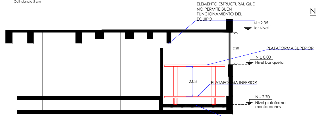
SECCIÓN 4-4" ESC 1:100
