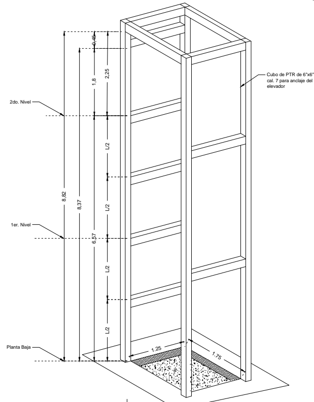
ISOMETRICO DE PTR
