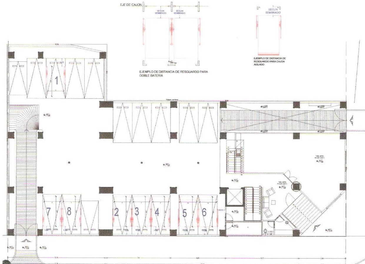
PLANTA BAJA
