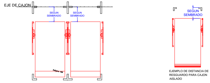
EJEMPLO DE DISTANCIA DE RESGUARDO PARA DOBLE BATERIA
