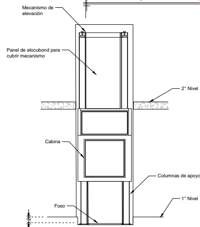
ALZADO (ESTRUCTURA)
