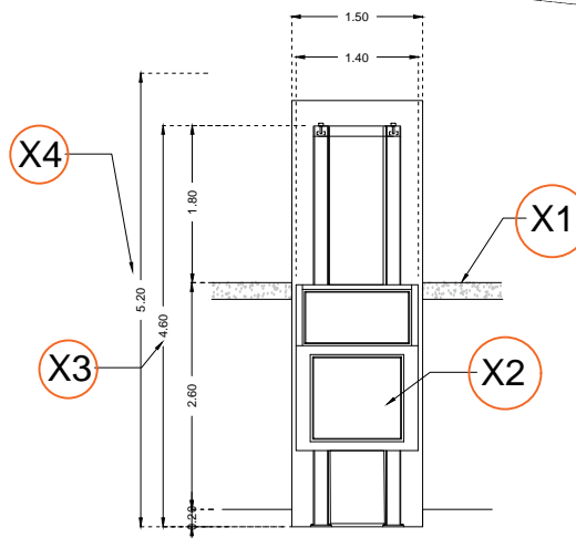
ALZADO (RECORRIDO)
