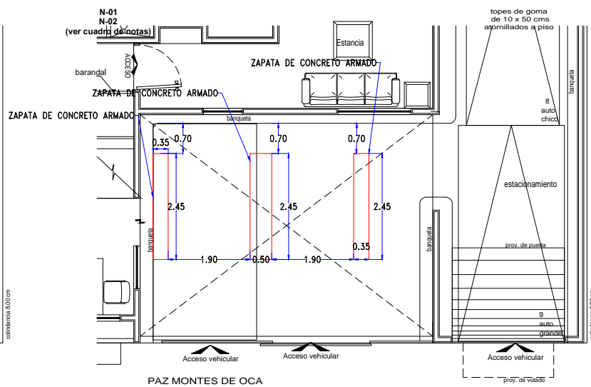
PLANTA BAJA
