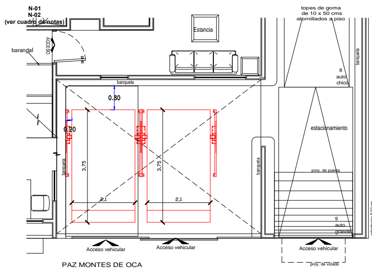
PLANTA BAJA
