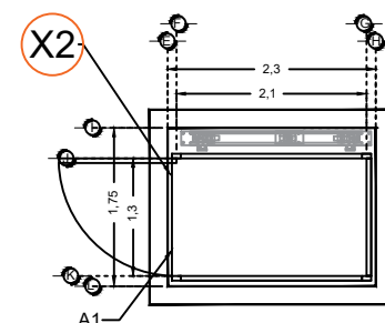
DIMENSIONES DE CABINA
