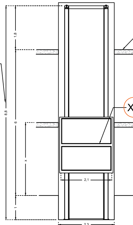
ALZADO (RECORRIDO)
