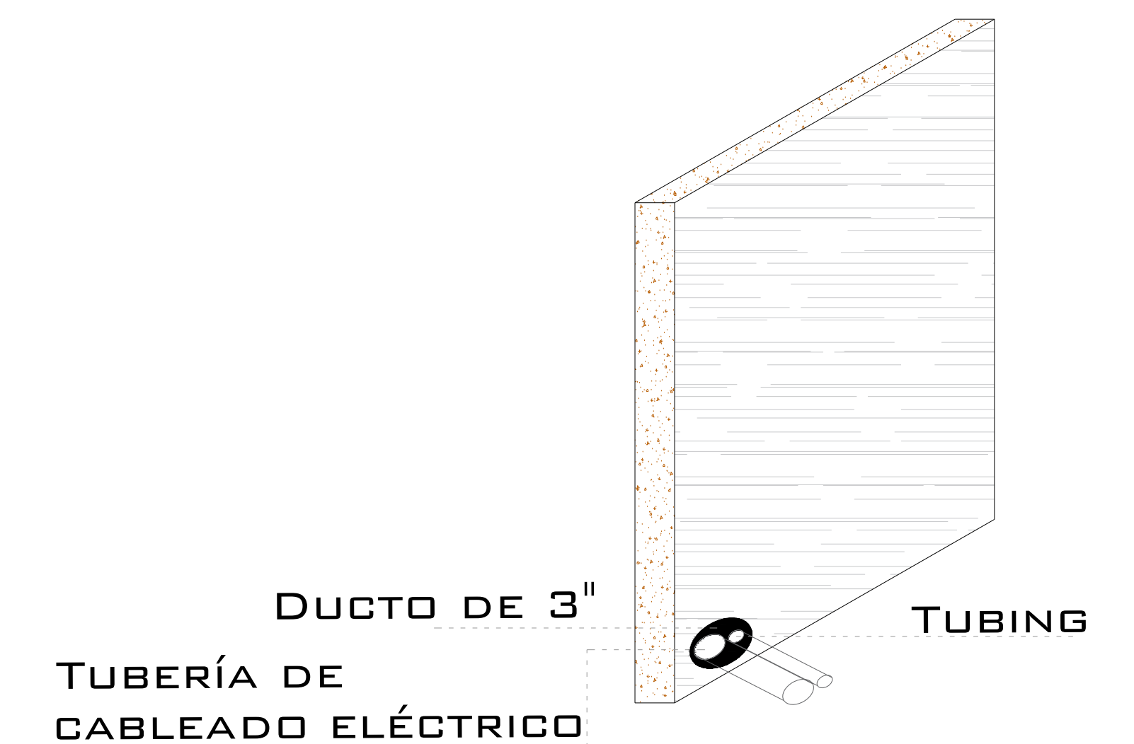
DUCTO DE ALIMENTACION ISOMETRICO
