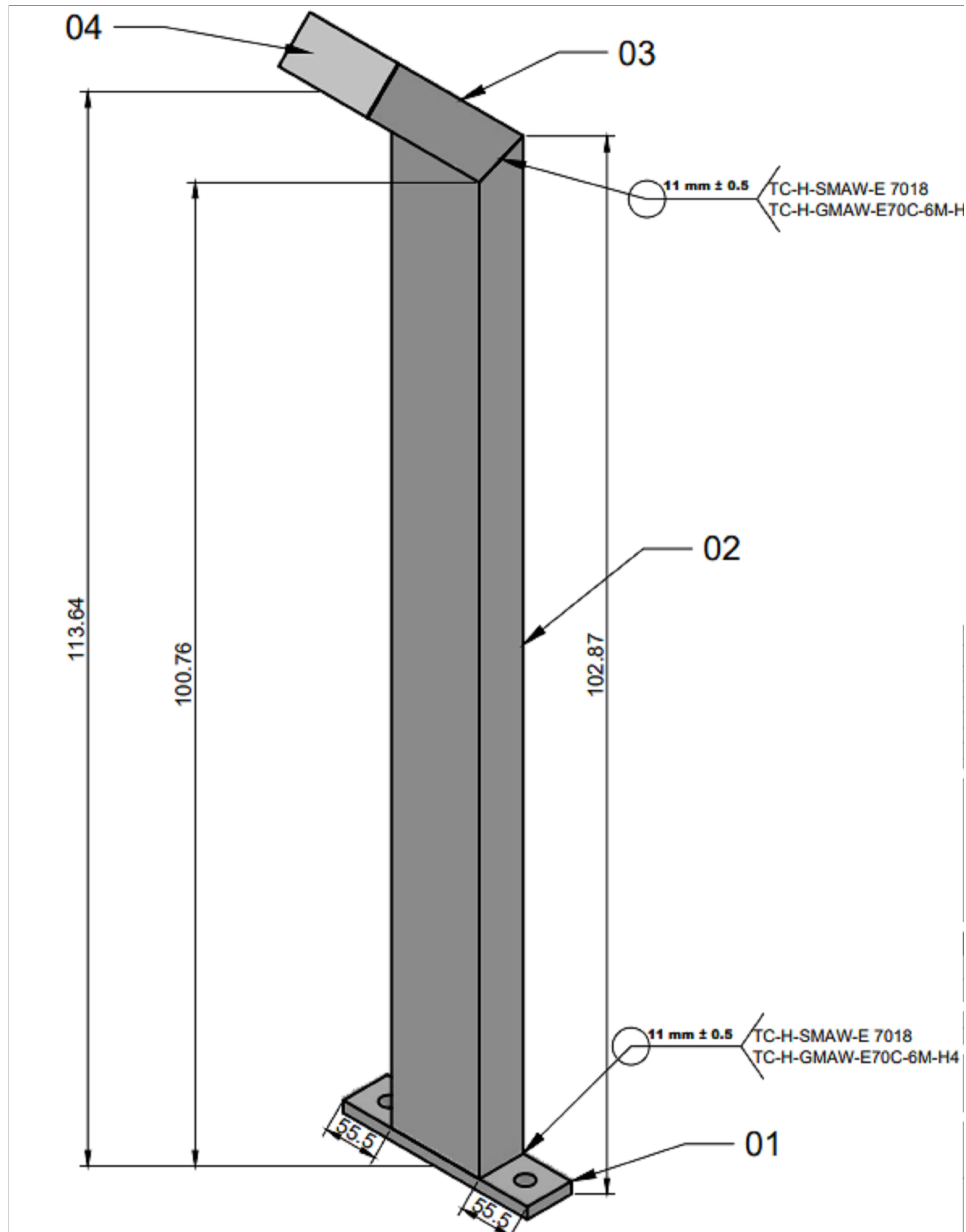
BOTONERA EN PEDESTAL
