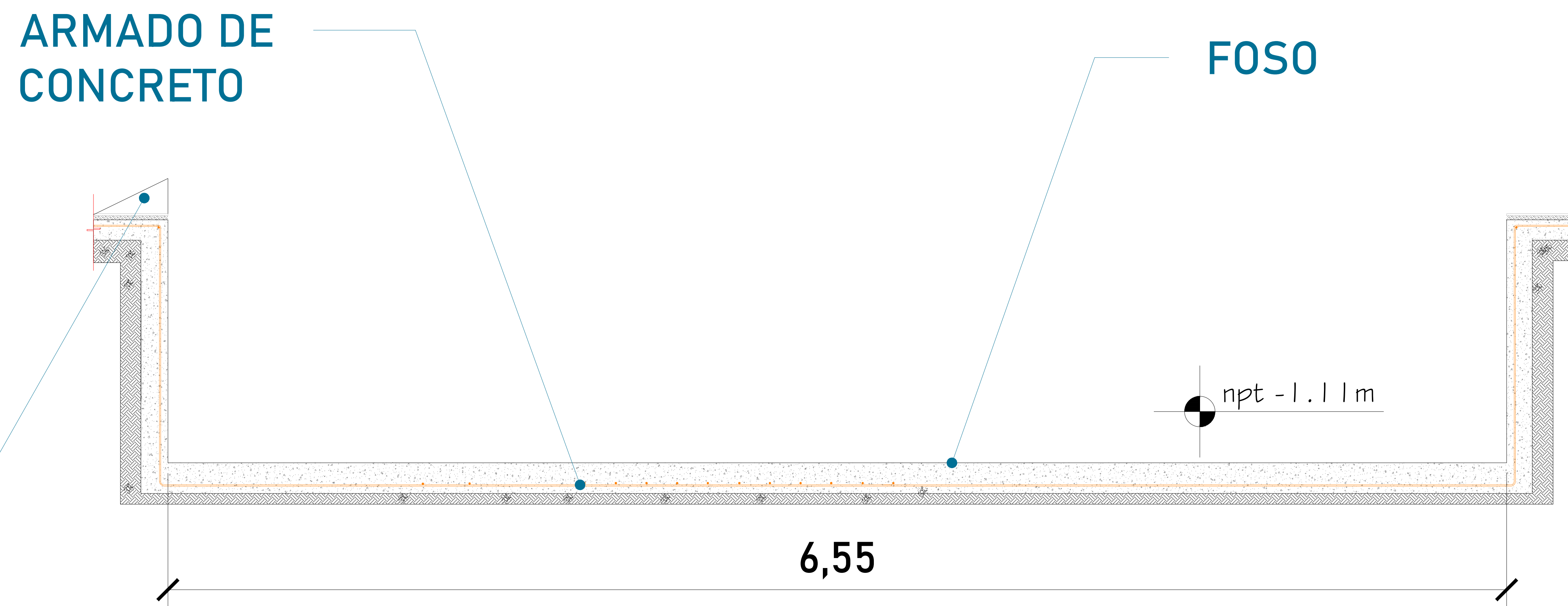
FOSO (VISTA LATERAL)
