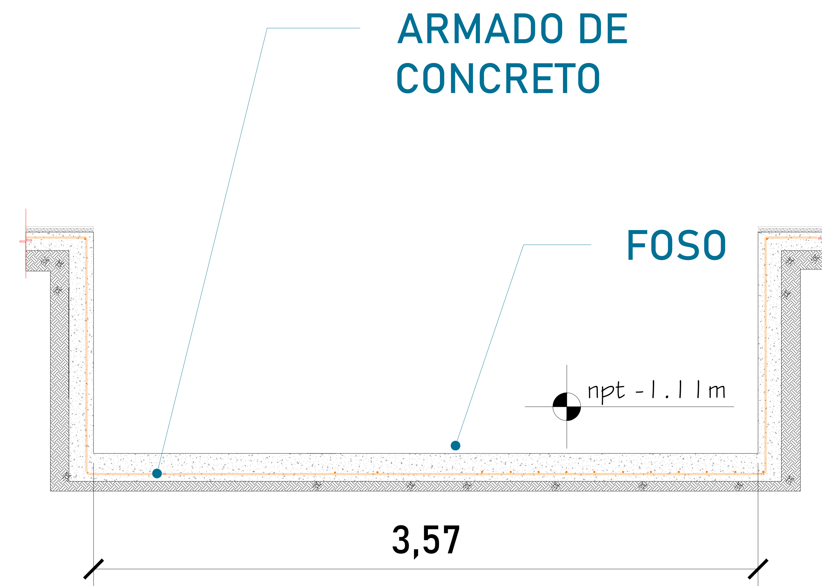
FOSO (VISTA FRONTAL)
