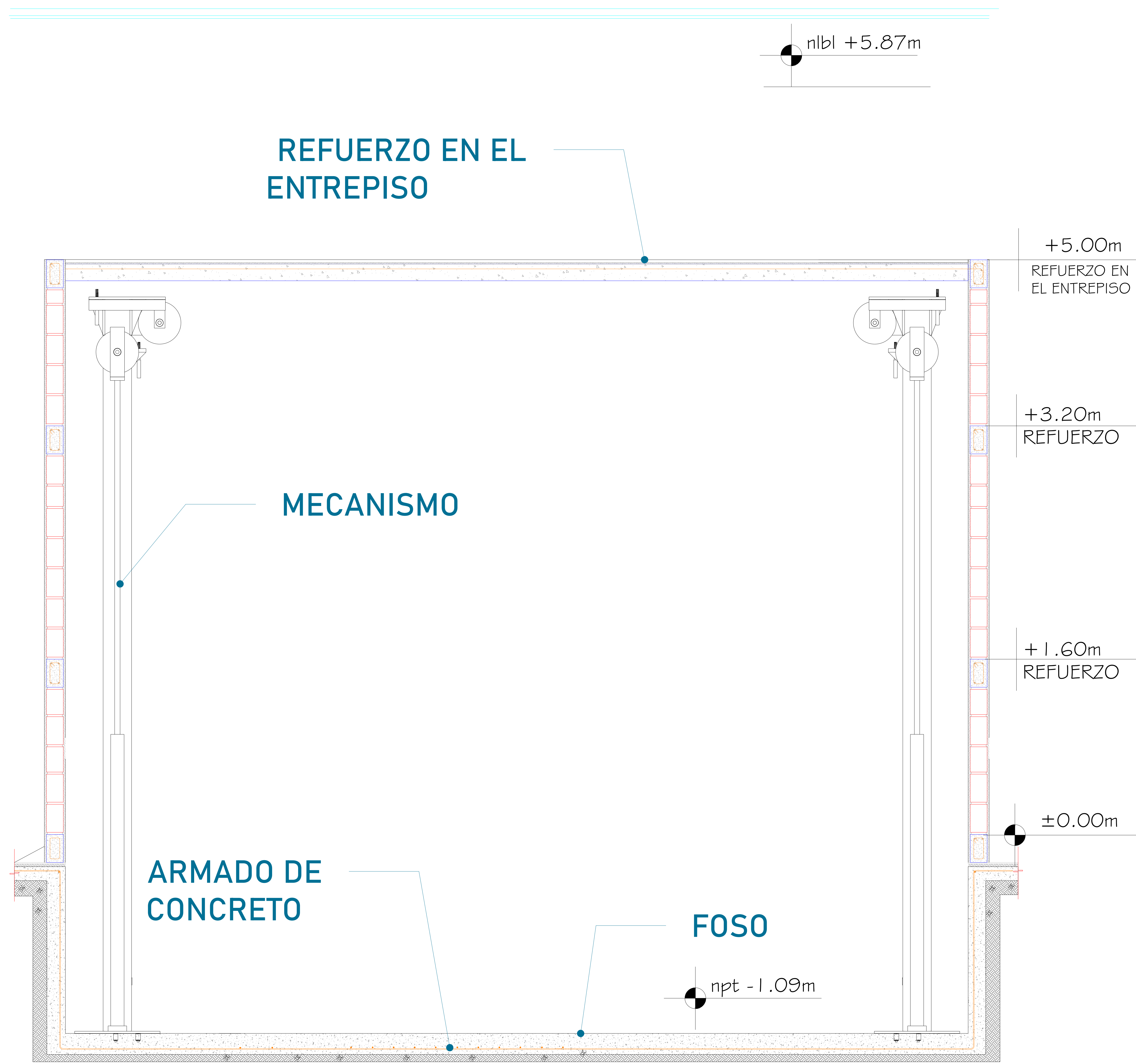
FOSO (VISTA LATERAL)
