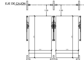
EJEMPLO DE DISTANCIA DE RESGUARDO PARA DOBLE BATERIA
