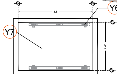
FOSO VISTA PLANTA
