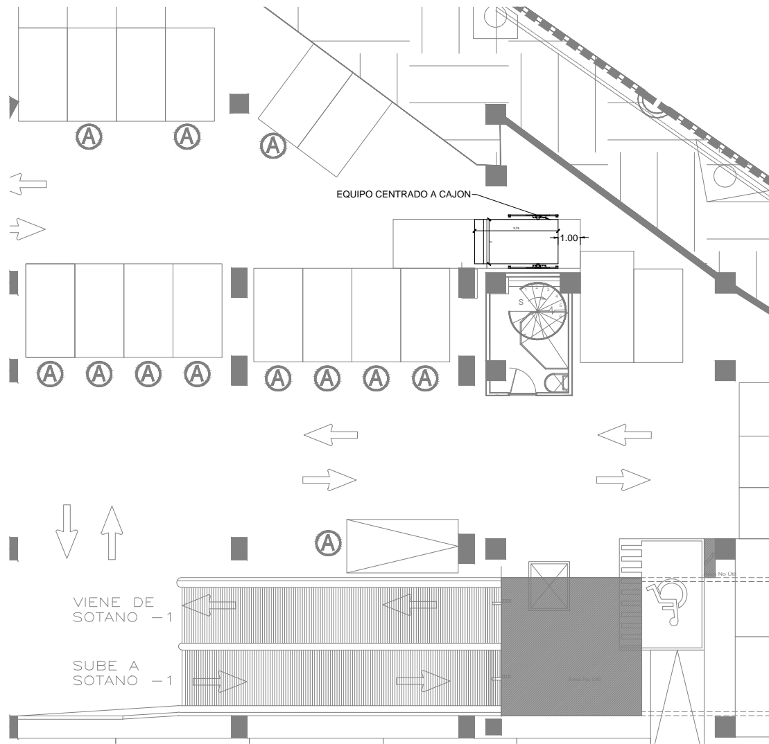
EJEMPLO DE DISTANCIA DE RESGUARDO PARA CAJON ASILADO
