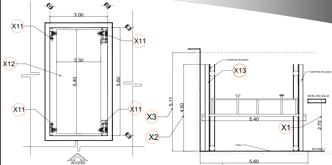
ALZADO (RECORRIDO)
