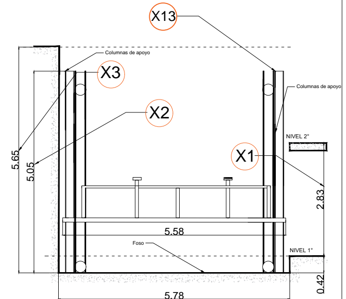
ALZADO (RECORRIDO)
