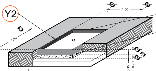
FOSO-VISTA ISOMETRICO
