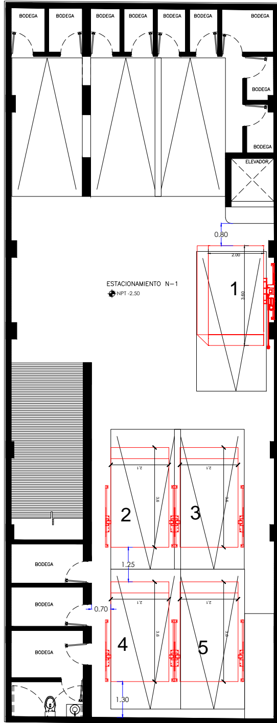
ARQ-01 PLANTA ESTACIONAMIENTO N-1 ESCALA 1:50
