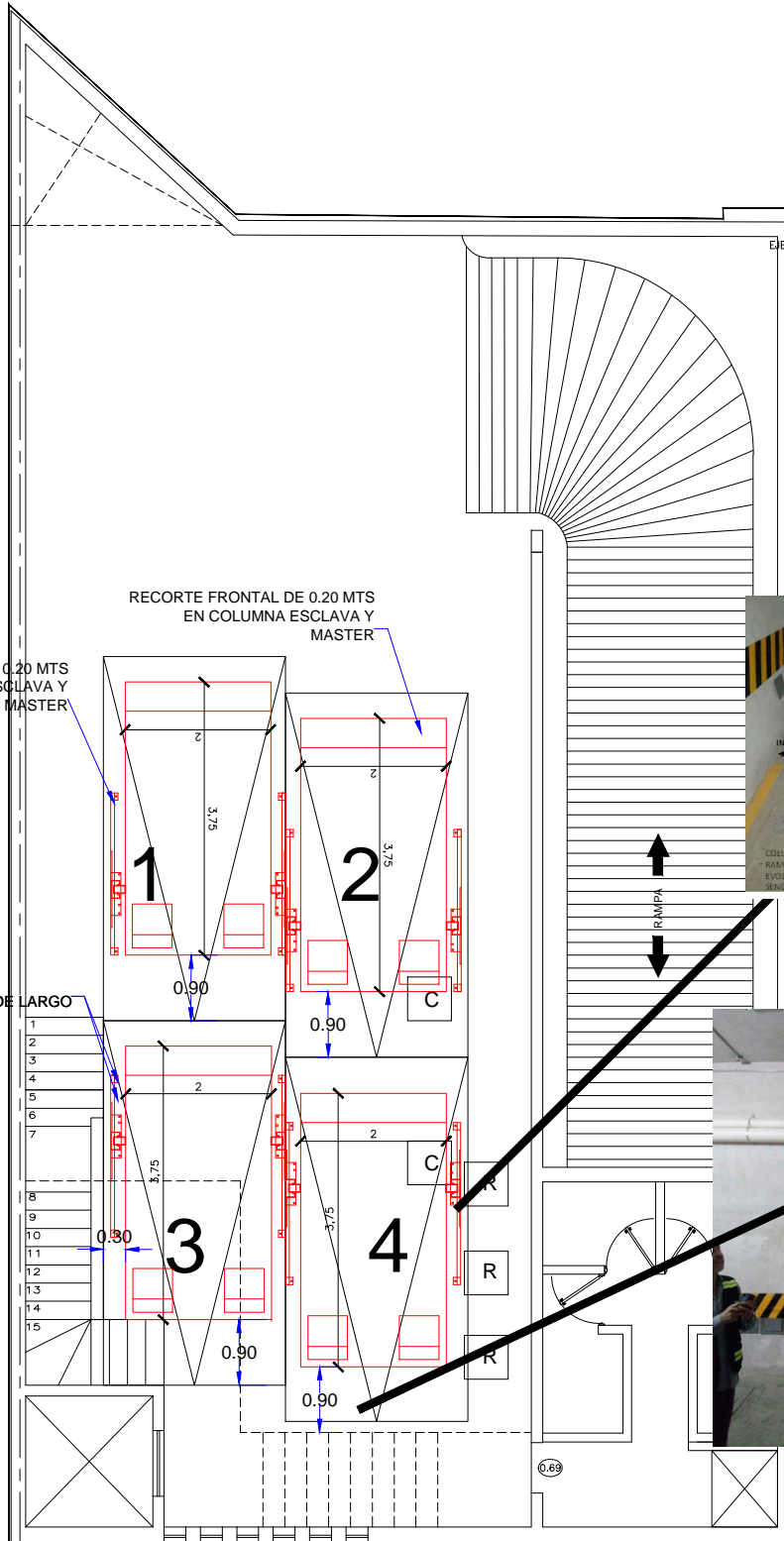
PLANTA SEMISOTANO
