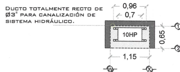
DESCRIPCION DE UNIDAD HIDRAULICA GABINETE (VISTA PLANTA)
