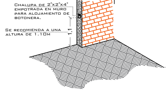
BOTONERA EMPOTRADA
