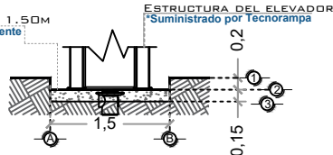
FOSO DEL ELEVADOR VISTA FRONTAL
