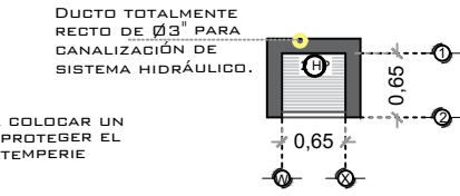
DESCRIPCION DE UNIDAD HIDRAULICA GABINETE (VISTA PLANTA)
