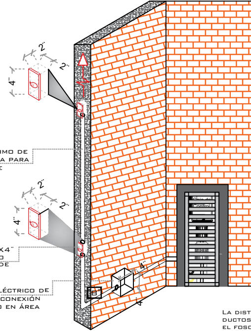
ESPECIFICACIONES ELECTRICAS
