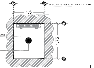
FOSO DEL ELEVADOR VISTA PLANTA
