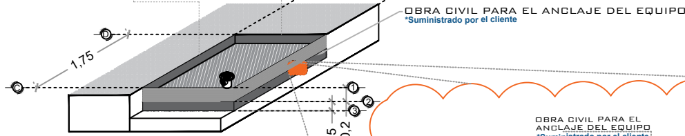
FOSO DEL ELEVADOR ISOMETRICO
