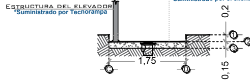
FOSO DEL ELEVADOR VISTA LATERAL
