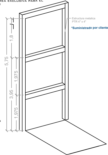
REFUERZO DE ANCLAJE ALTURAS
