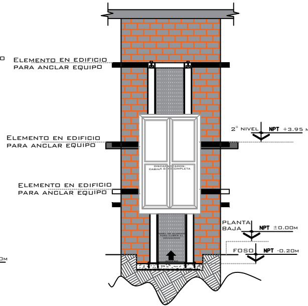
ELEVADOR SEMICOMPLETA FRONTAL
