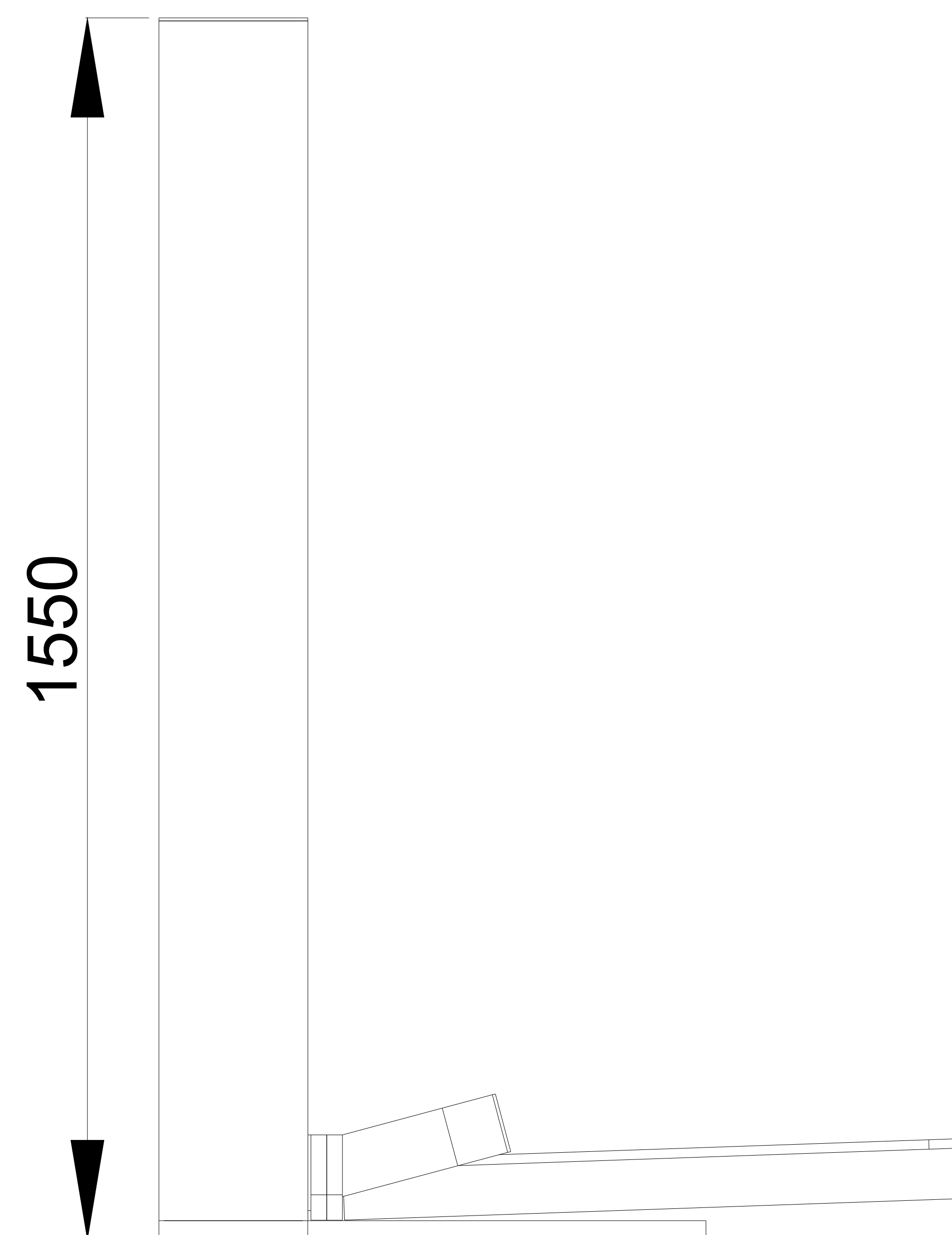
VISTA LATERAL
