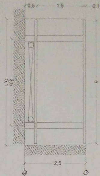
CORTE DE UNDER RAMP (Altura de foso 2.50m)
