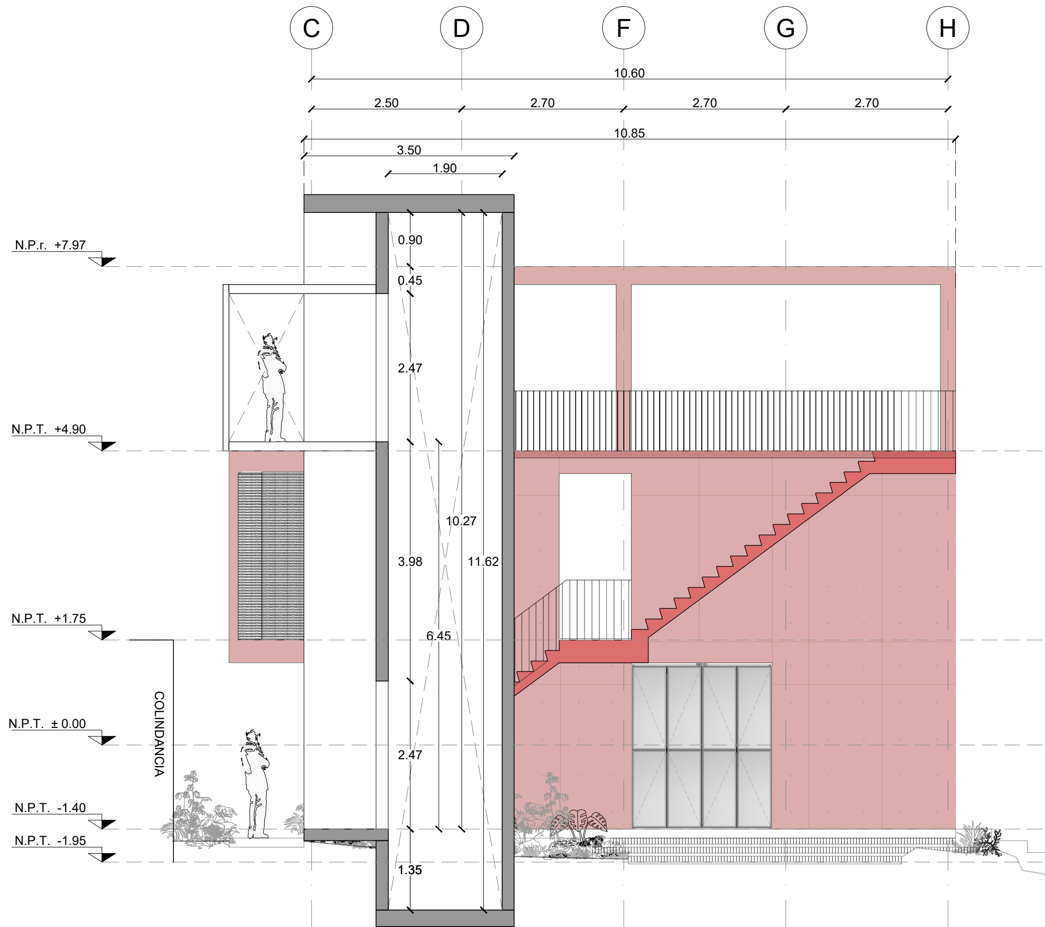
CORTE PROPUESTA ELEVADOR AMPLIACIÓN HCA
