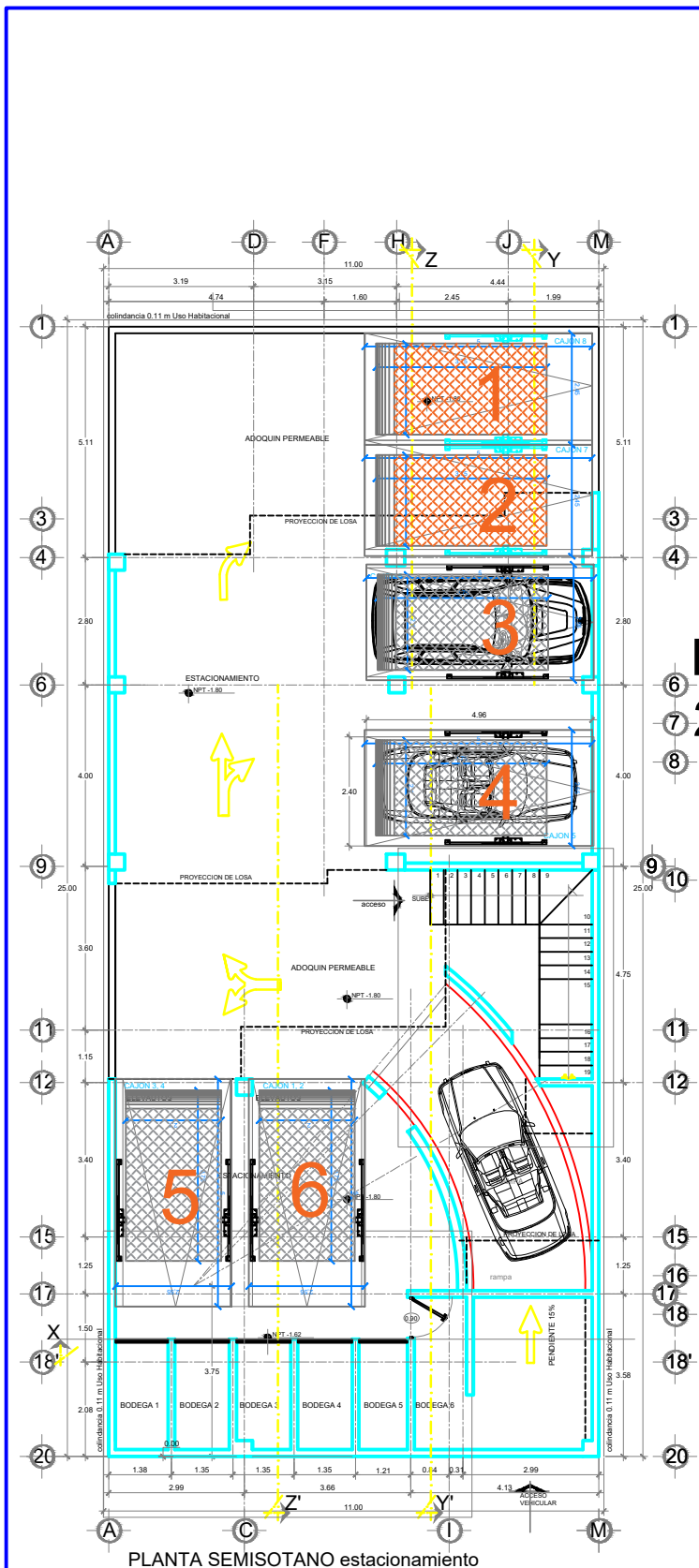
PLANTA SEMISOTANO estacionamiento
