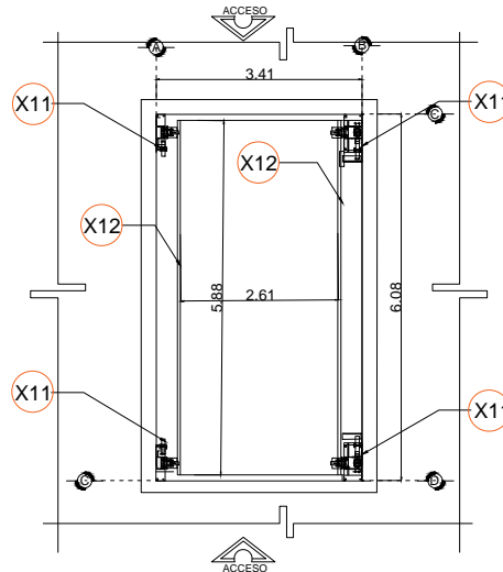
FOSO VISTA PLANTA
