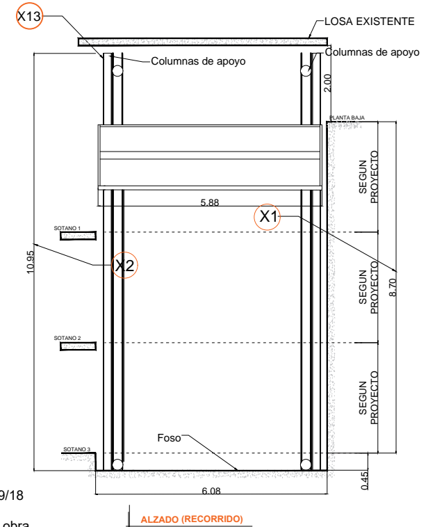
ALZADO (RECORRIDO)
