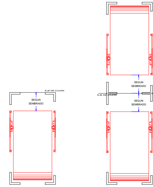
INSTALACION DE RAMPAS CENTRADAS A CAJON
