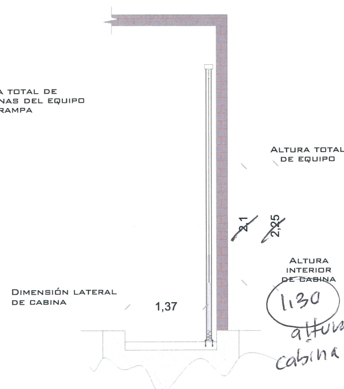
ALTURA DE CABINA SEMICOMPLETA
