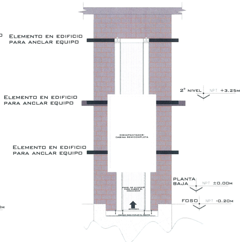
ELEVADOR SEMICOMPLETA FRONTAL
