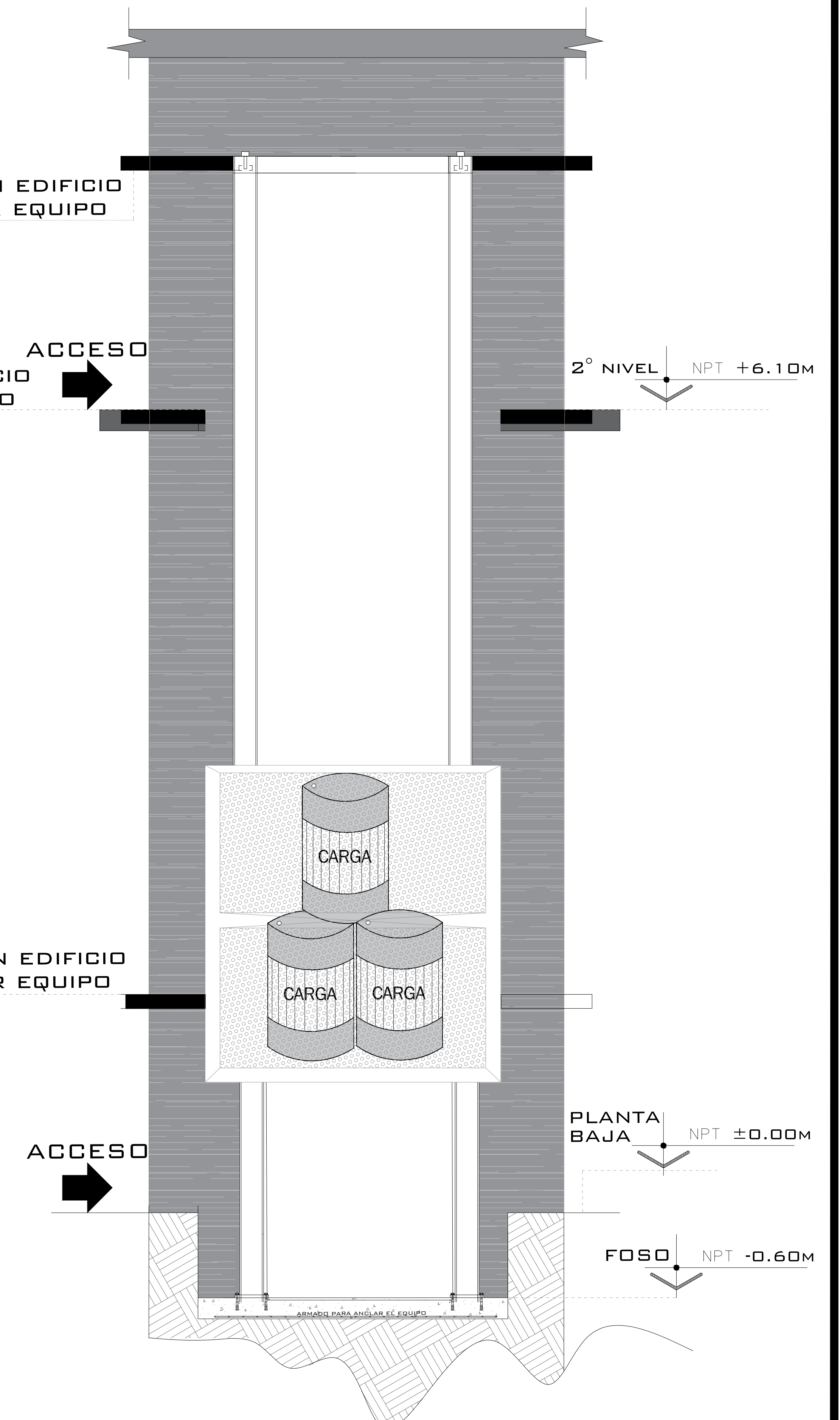
ELEVADOR TIPO CARGA LATERAL
