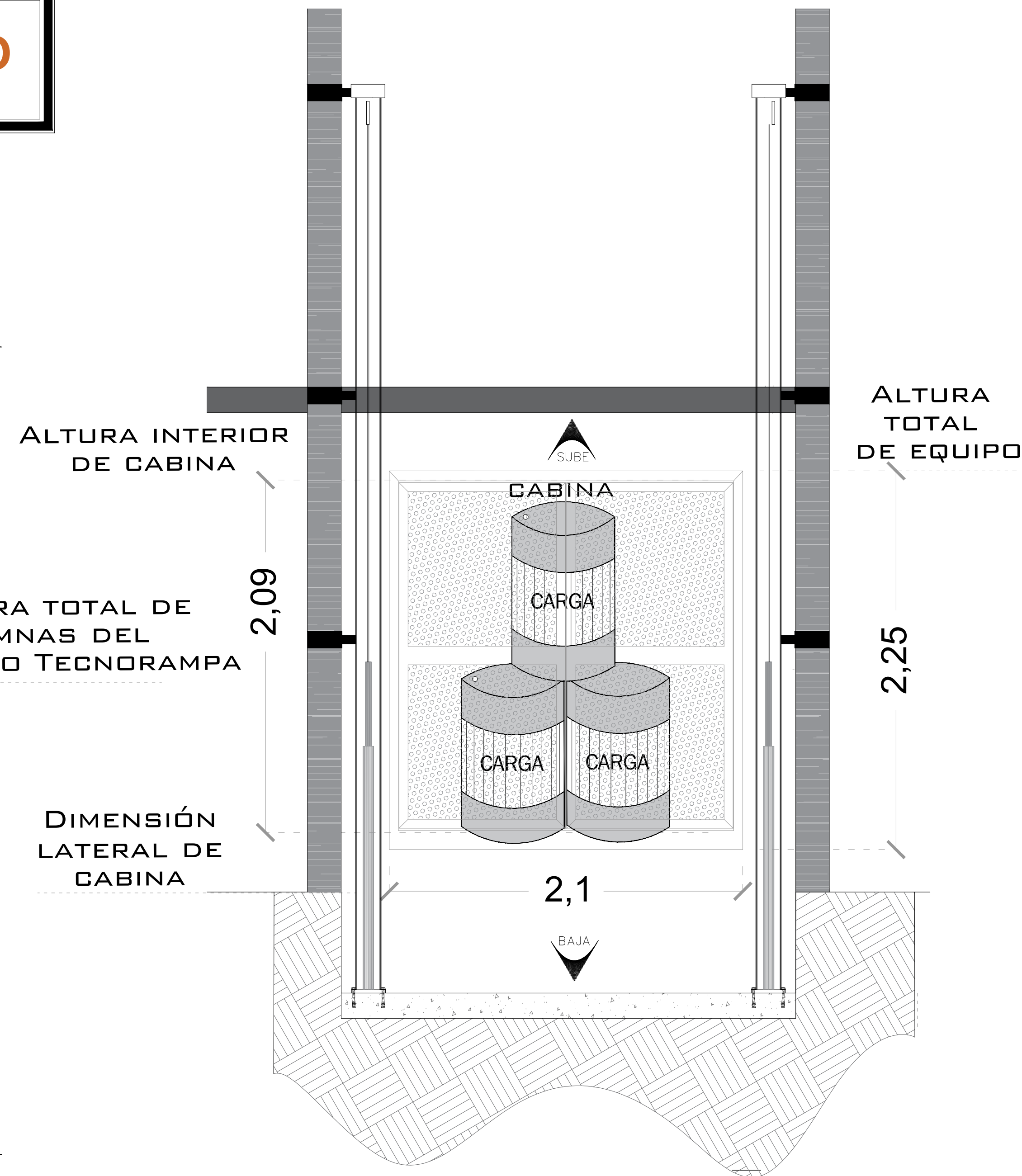
ALTURA DE CABINA TIPO CARGA
