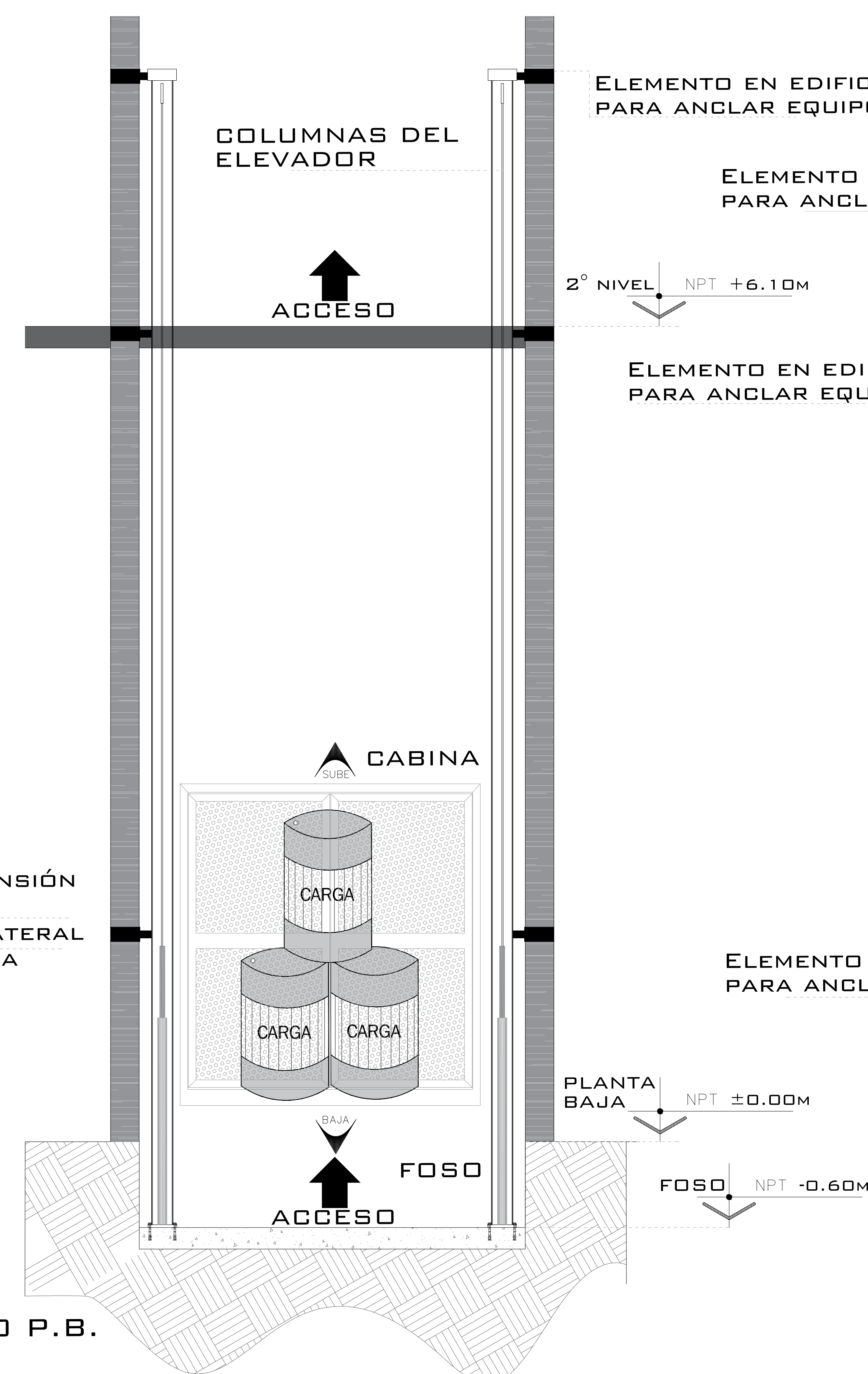
ELEVADOR TIPO CARGA FRONTAL
