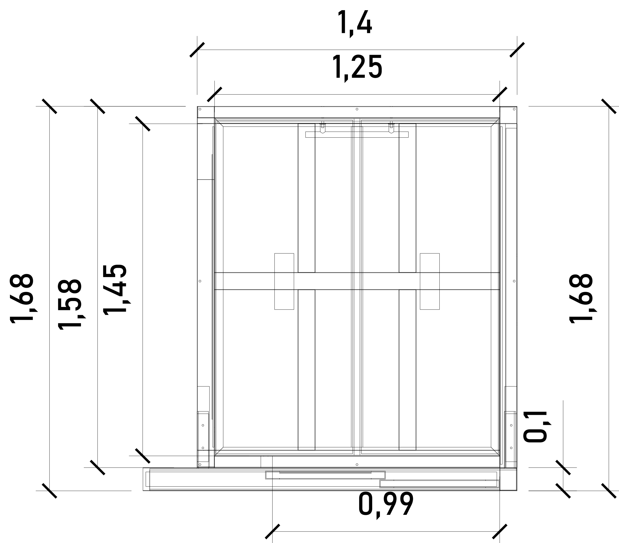
CABINA (VISTA EN PLANTA)
