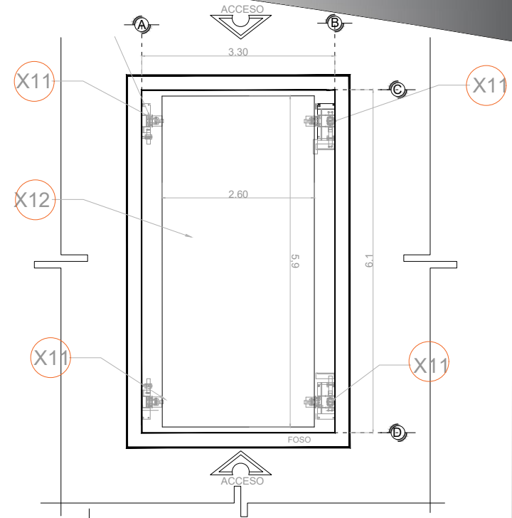
FOSO VISTA PLANTA
