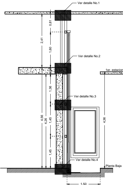
Corte Esquemático (ESTRUCTURA)
