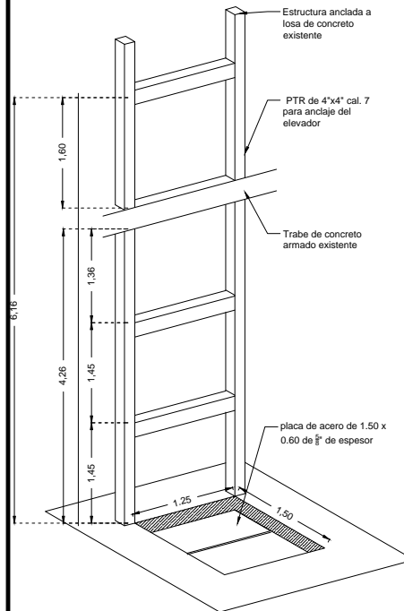
REQUERIMIENTOS DE REFUERZO (ESTRUCTURA)
