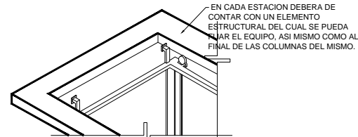
DETALLE DE FIJACION
