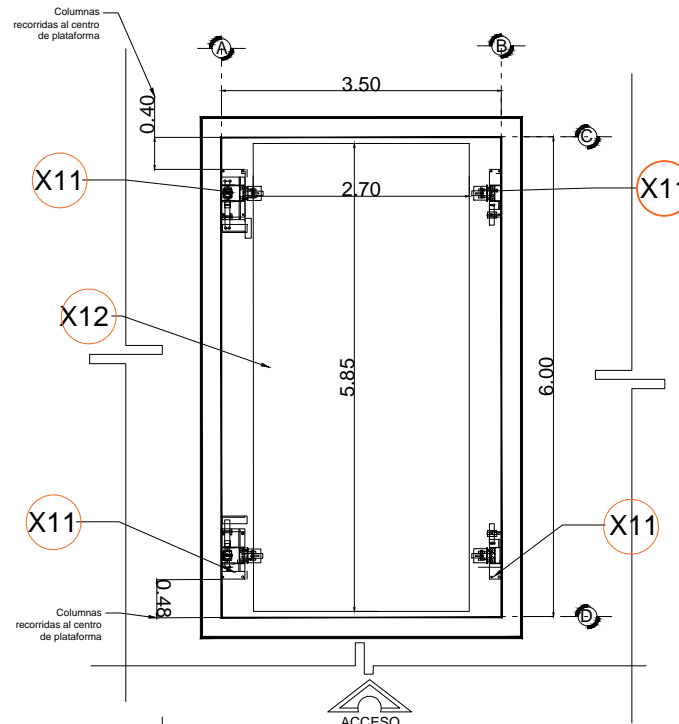
FOSO VISTA PLANTA
