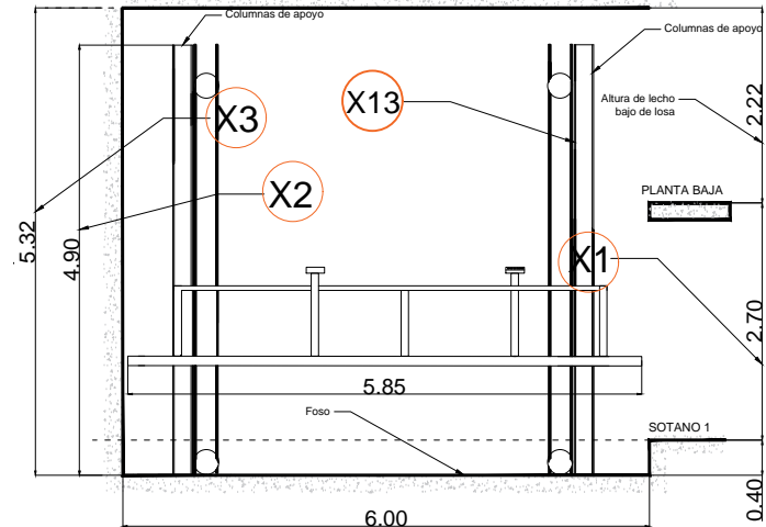
ALZADO (RECORRIDO)
