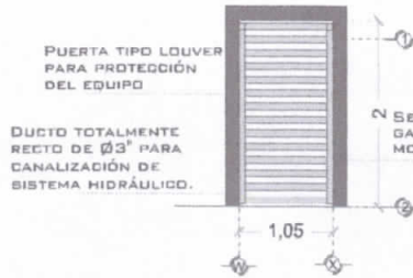
DESCRIPCIÓN DE UNIDAD HIDRÁULICA GABINETE (VISTA FRONTAL)
