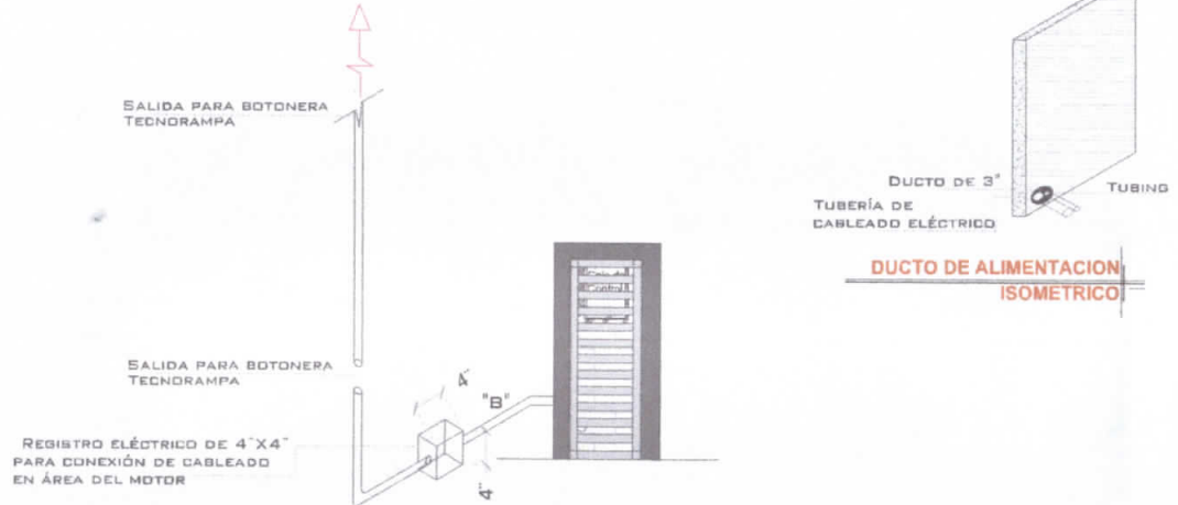
ESPECIFICACIONES ELECTRICAS
