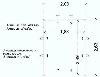
VISTA DEL ELEVADOR FRONTAL
