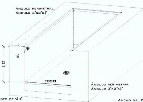
FOSO DEL ELEVADOR VISTA FRONTAL
