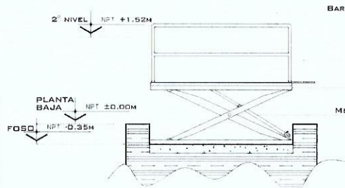
VISTA DEL ELEVADOR LATERAL
