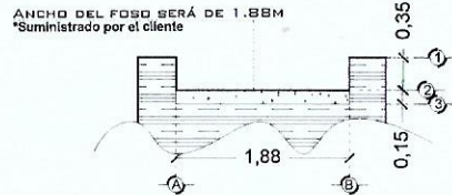
FOSO DEL ELEVADOR VISTA FRONTAL
