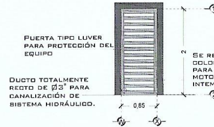
DESCRIPCIÓN DE UNIDAD HIDRAULICA GABINETE (VISTA FRONTAL)
