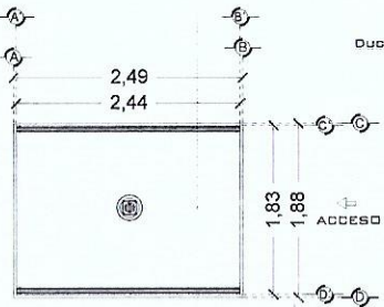
VISTA DEL ELEVADOR PLANTA
