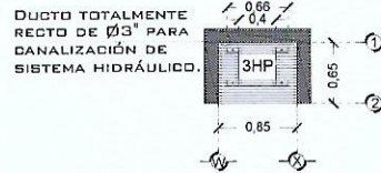
DESCRIPCIÓN DE UNIDAD HIDRAULICA GABINETE (VISTA PLANTA)
