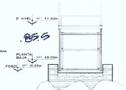
VISTA DEL ELEVADOR FRONTAL
