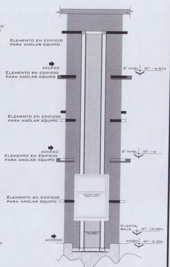
ELEVADOR MEDIA FRONTAL
