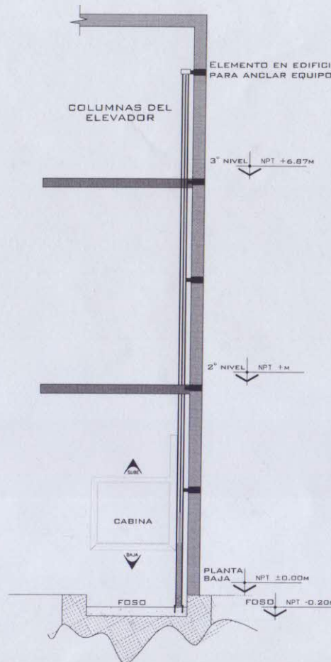
ELEVADOR MEDIA LATERAL
