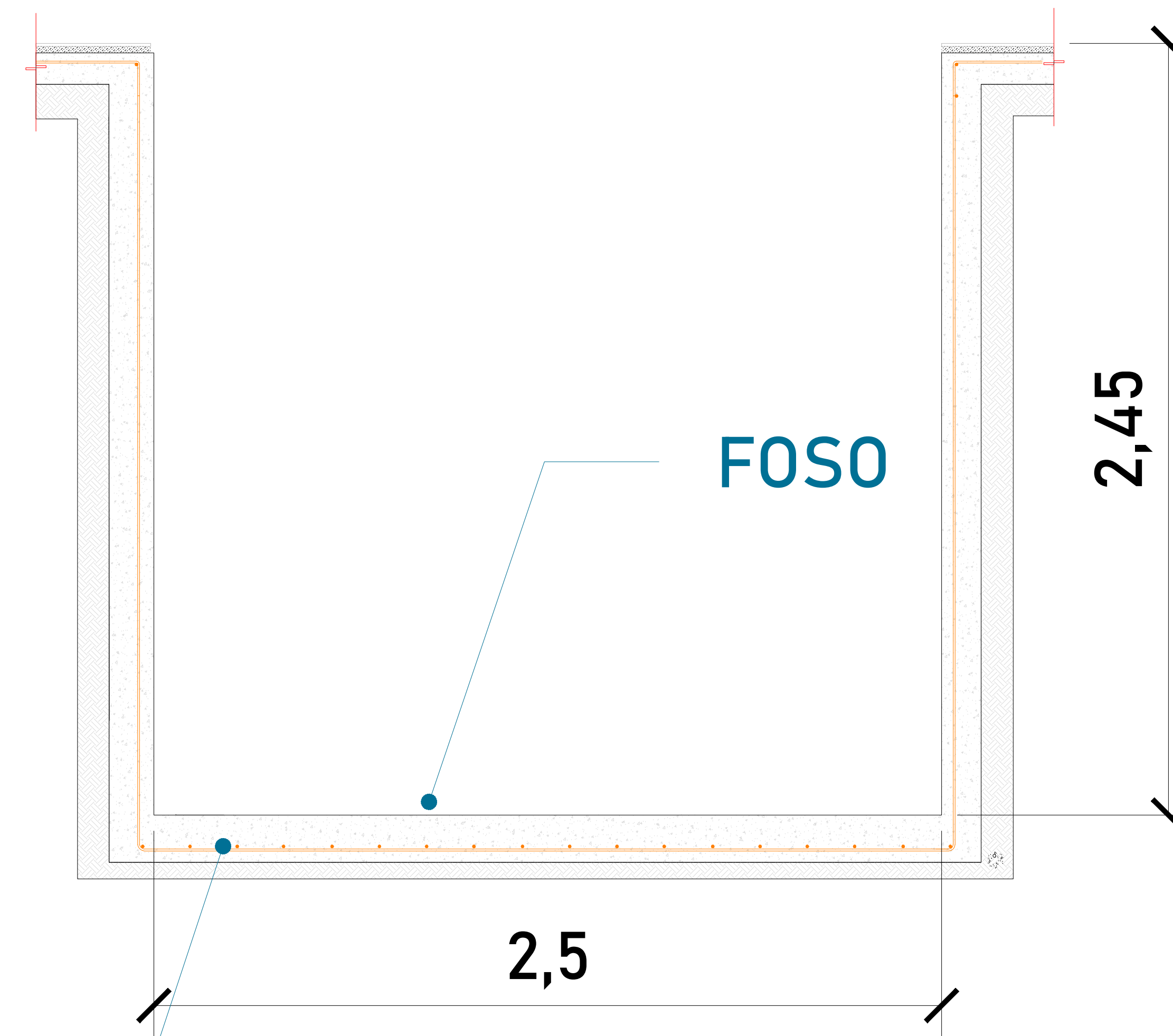
FOSO (VISTA FRONTAL)
