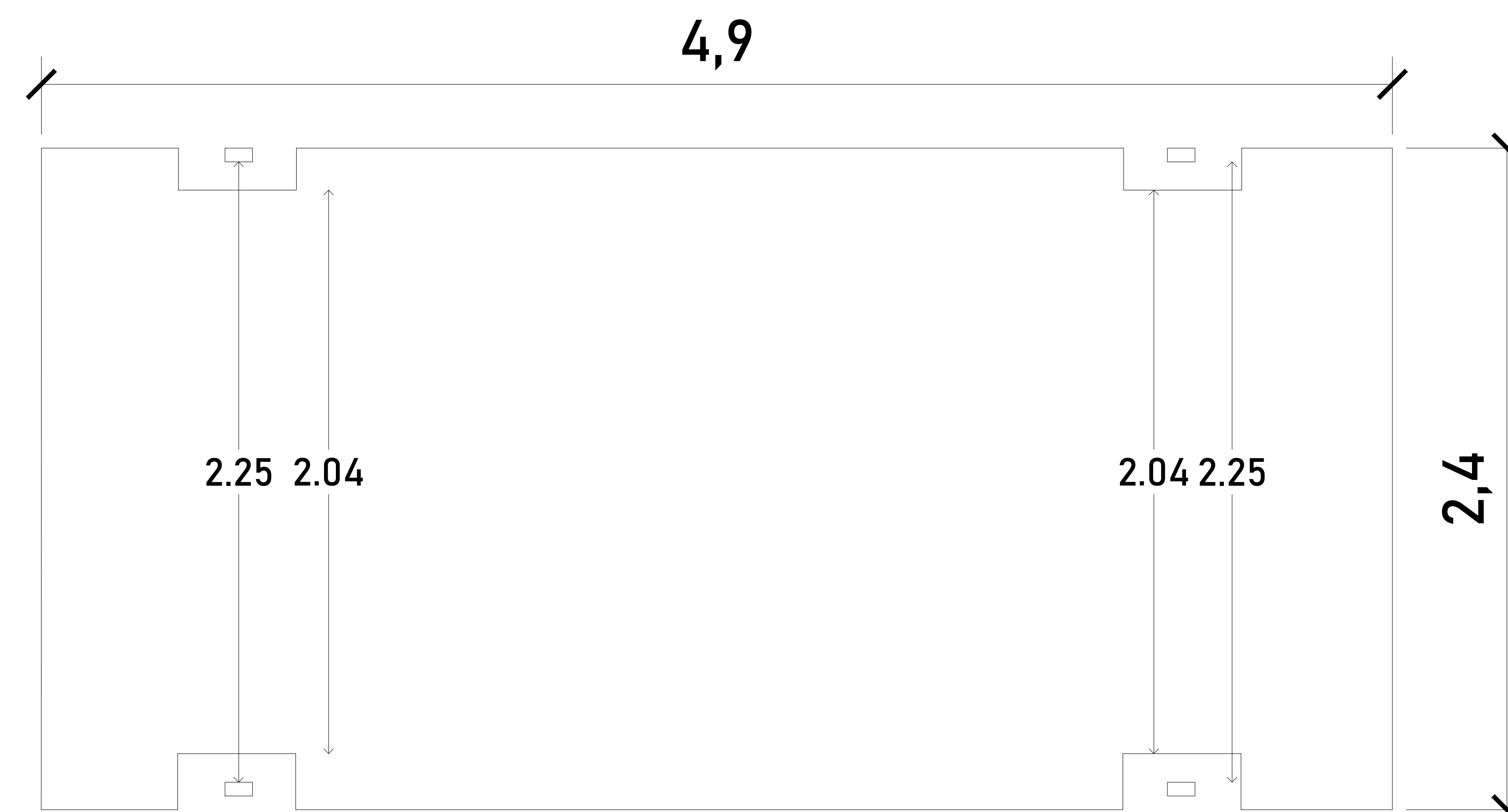
PLATAFORMA INFERIOR
