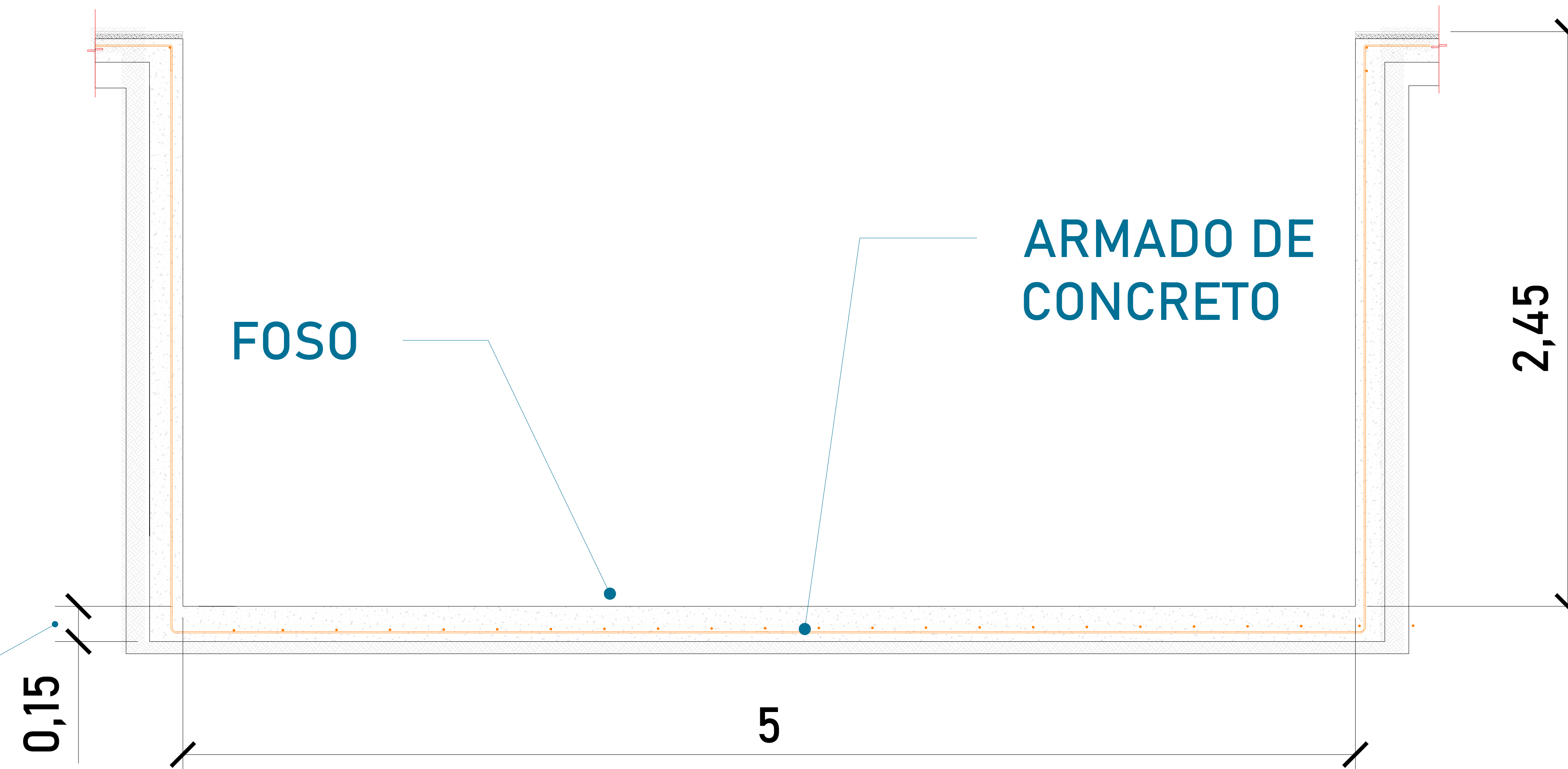
FOSO (VISTA LATERAL)
