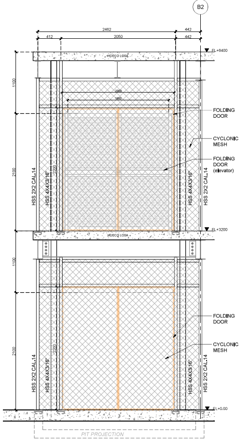
ELEVATION 1
