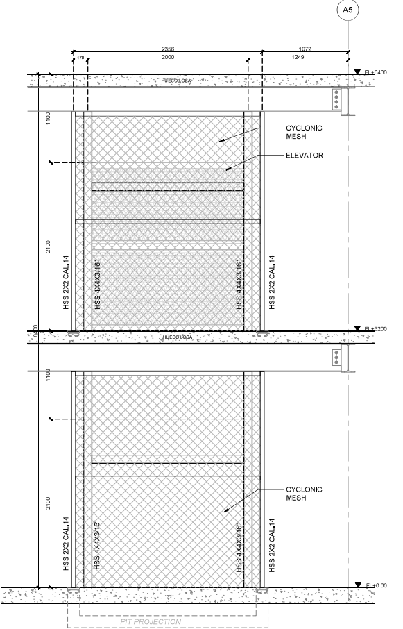
ELEVATION 2
