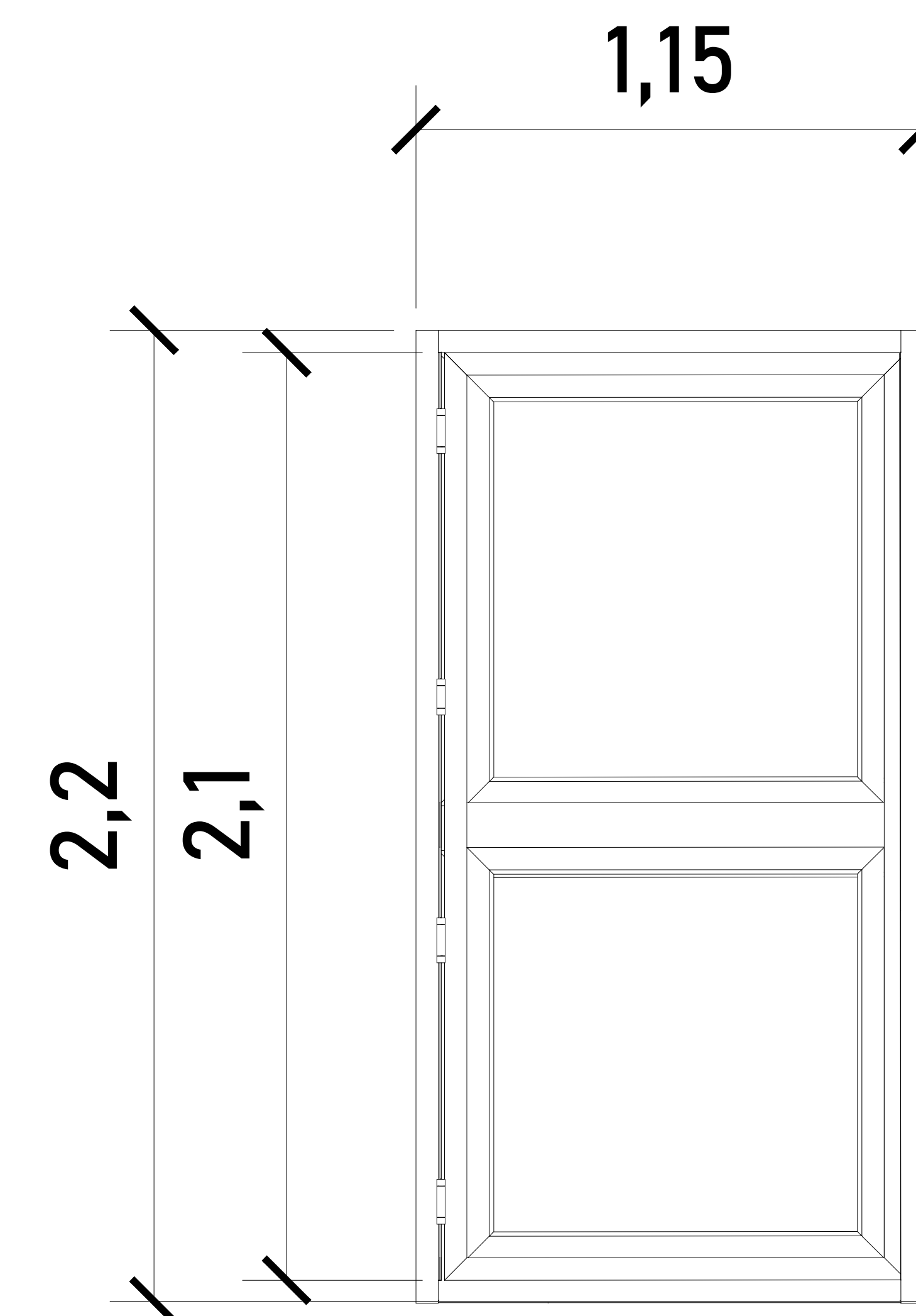
VISTA FRONTAL PUERTAS P.B. Y P.A.
