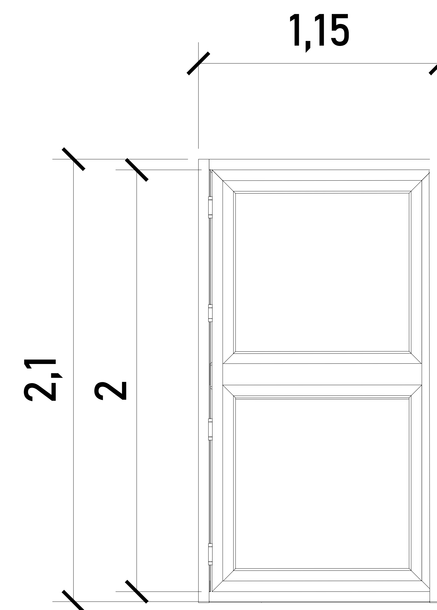
VISTA FRONTAL PUERTA P.2
