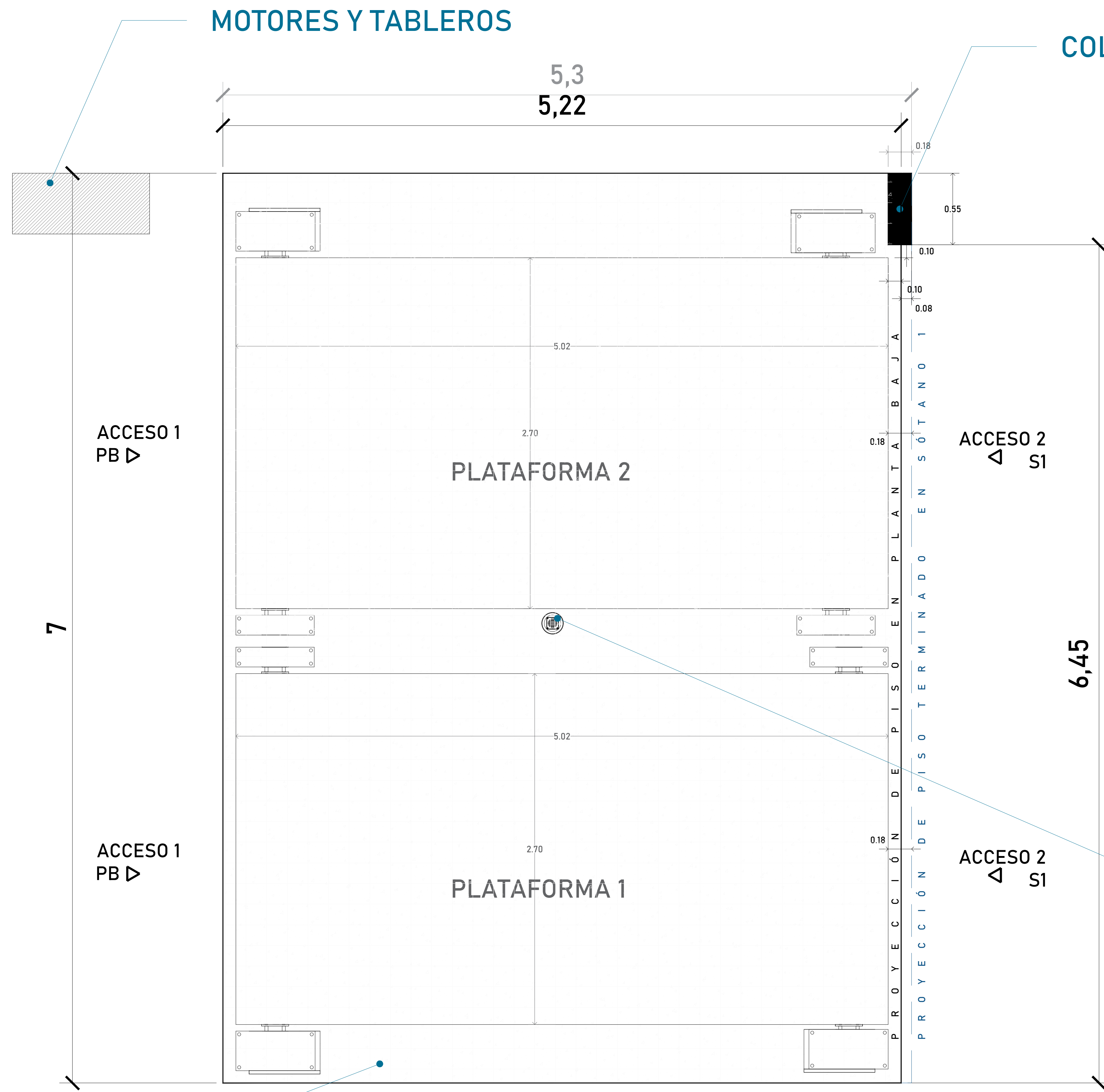
ARMADO (VISTA EN PLANTA)
