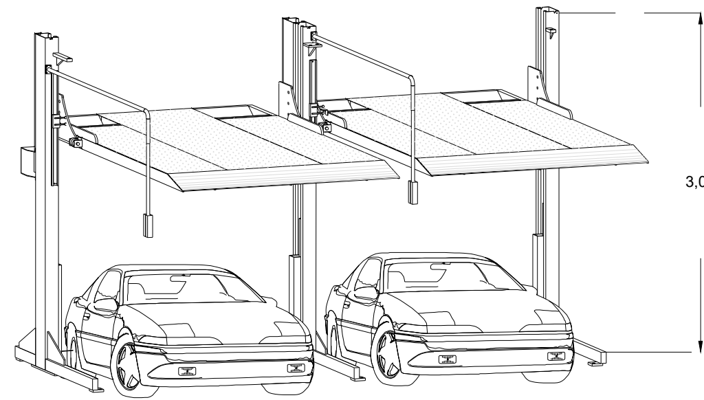
VISTA ISOMETRICO
