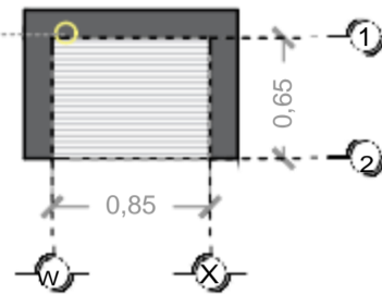
DESCRIPCION DE UNIDAD HIDRAULICA GABINETE (VISTA PLANTA)
