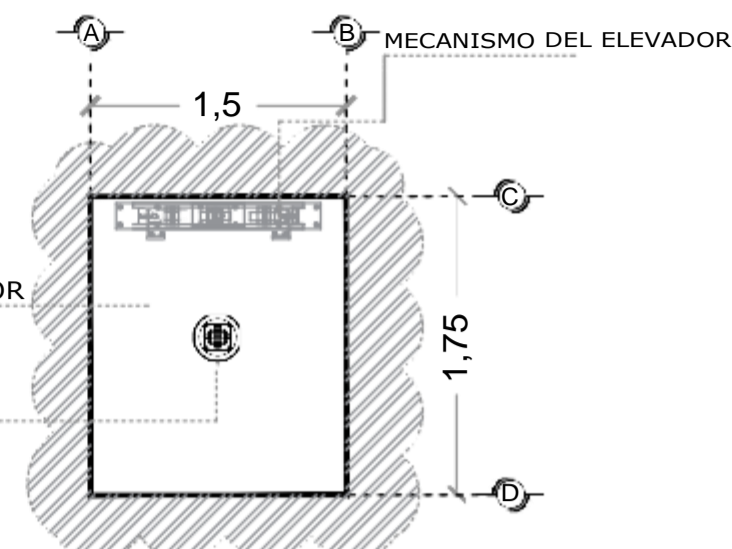
FOSO DEL ELEVADOR VISTA PLANTA
