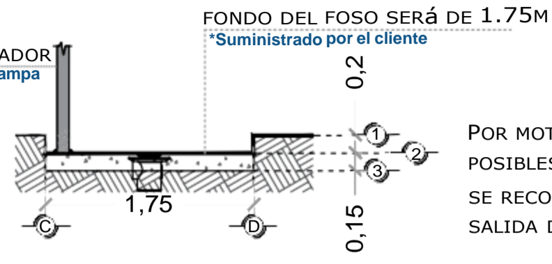
FOSO DEL ELEVADOR VISTA LATERAL
