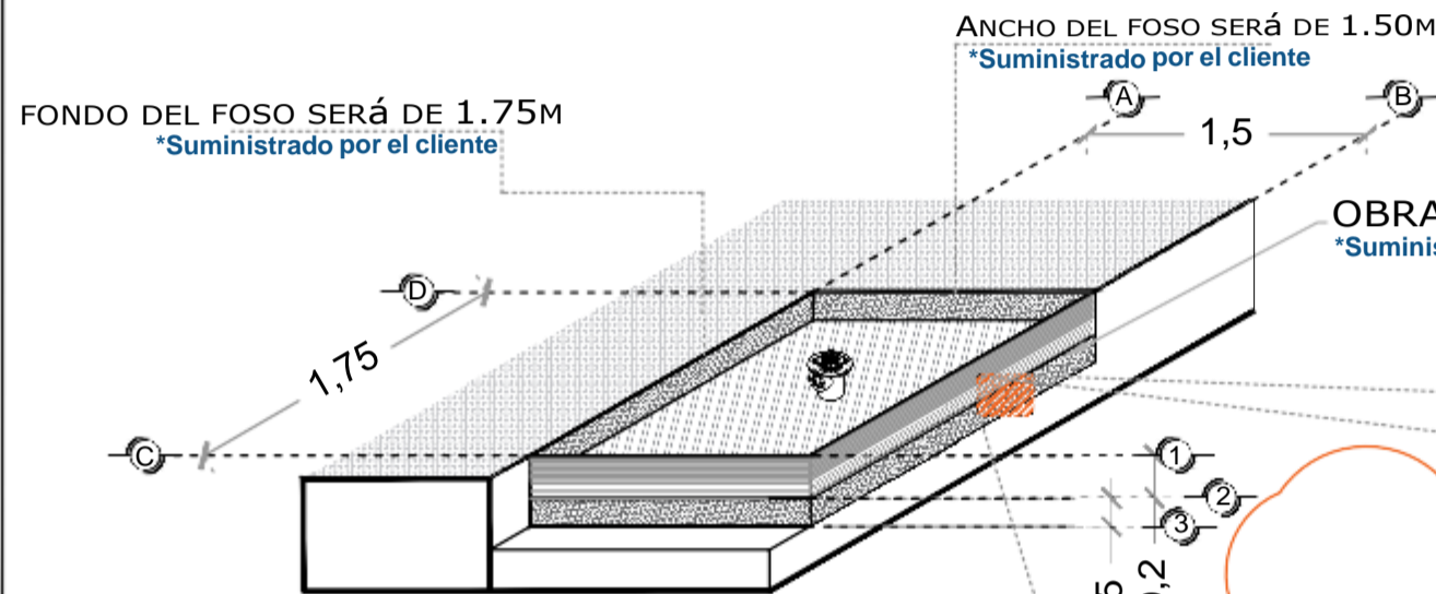
FOSO DEL ELEVADOR ISOMETRICO
