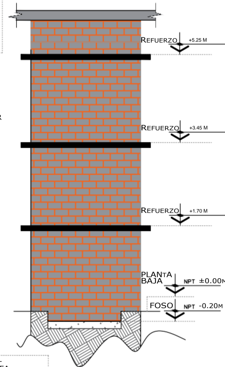
REFUERZO DE ANCLAJE ALTURAS
