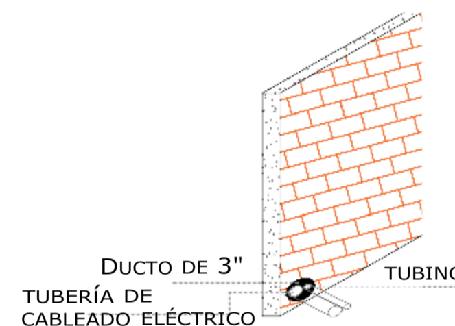
DUCTO DE ALIMENTACION ISOMETRICO
