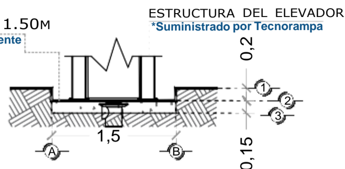
FOSO DEL ELEVADOR VISTA FRONTAL
