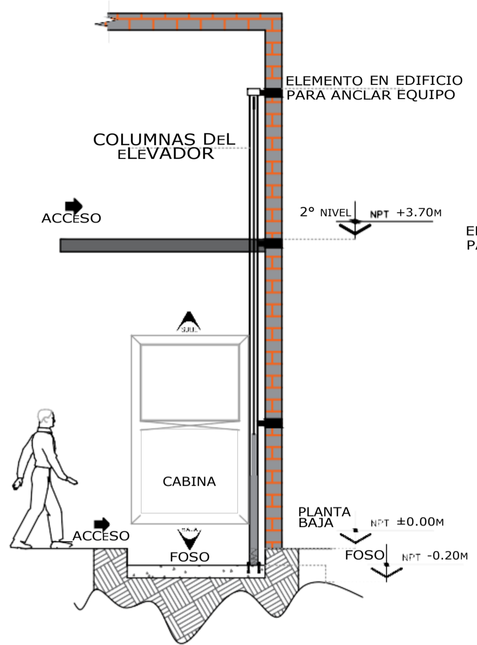
ELEVADOR SEMICOMPLETA LATERAL
