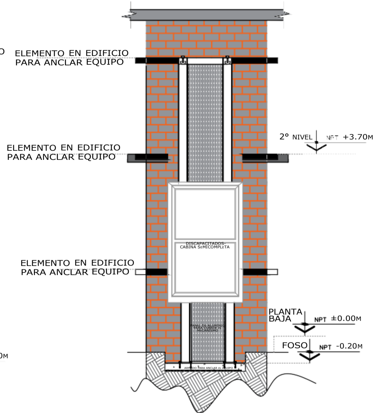
ELEVADOR SEMICOMPLETA FRONTAL
