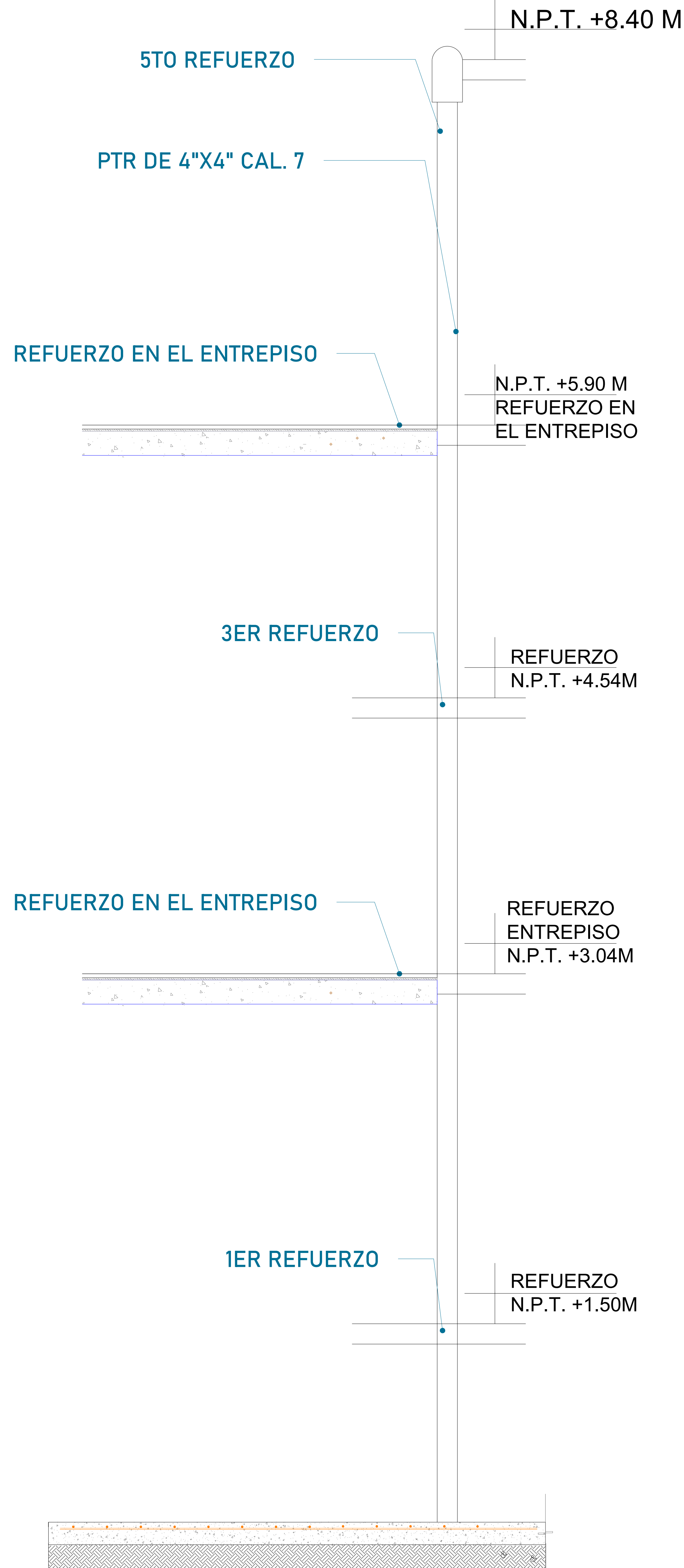
FOSO (VISTA LATERAL)
