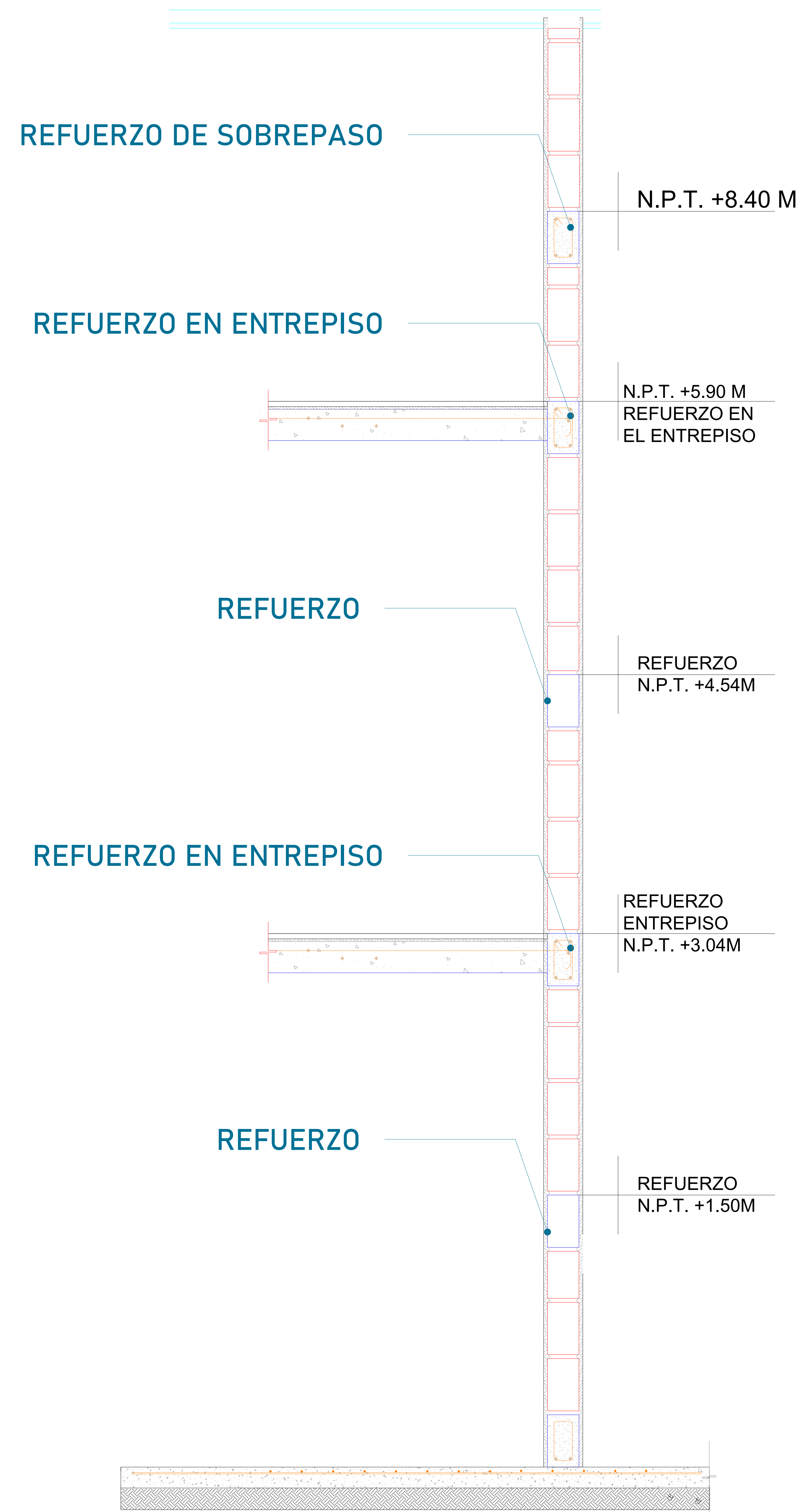
FOSO (VISTA LATERAL)
