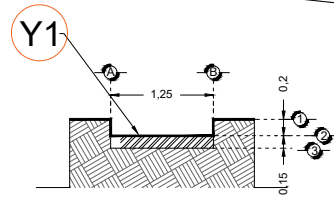
FOSO VISTA FRONTAL
