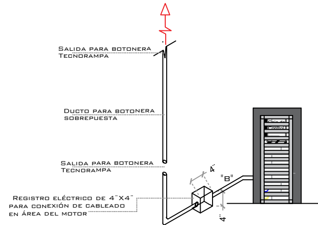
ESPECIFICACIONES ELECTRICAS
