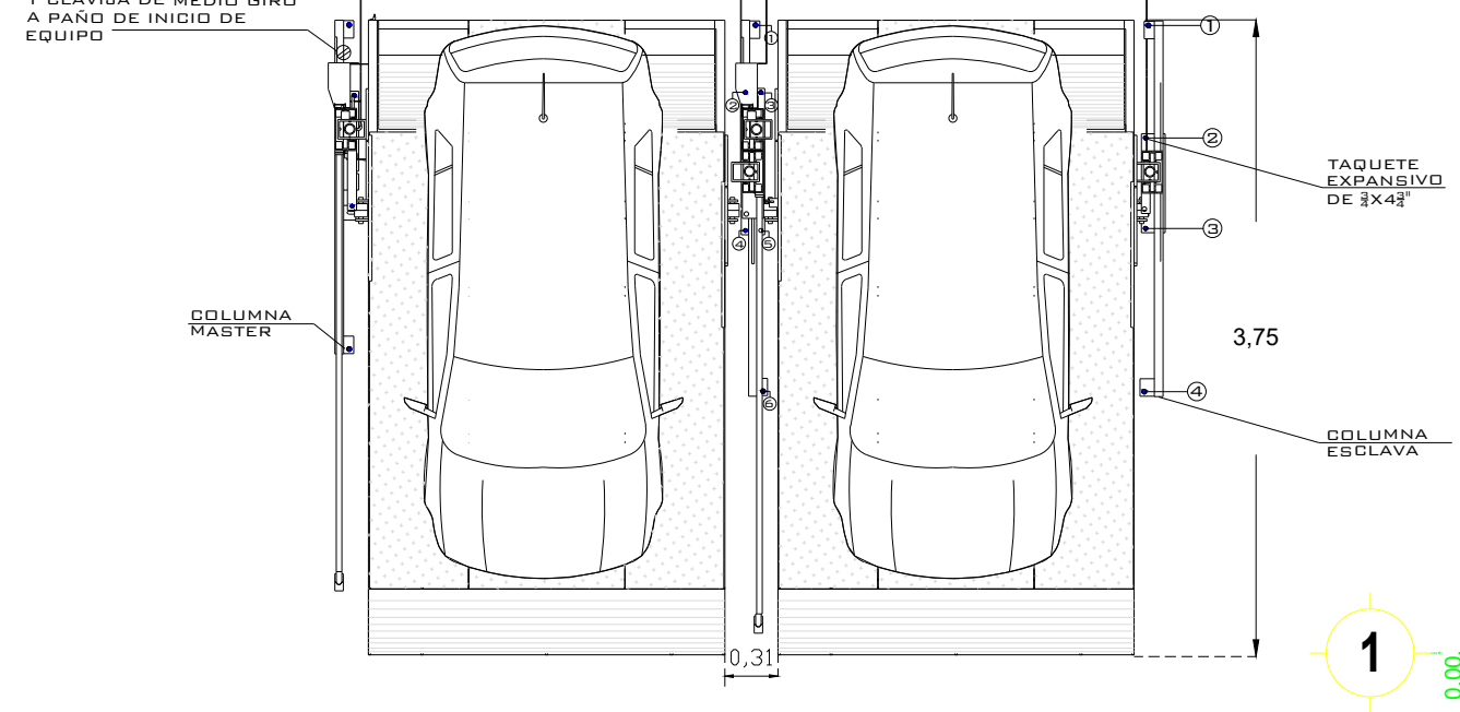
VISTA SUPERIOR
