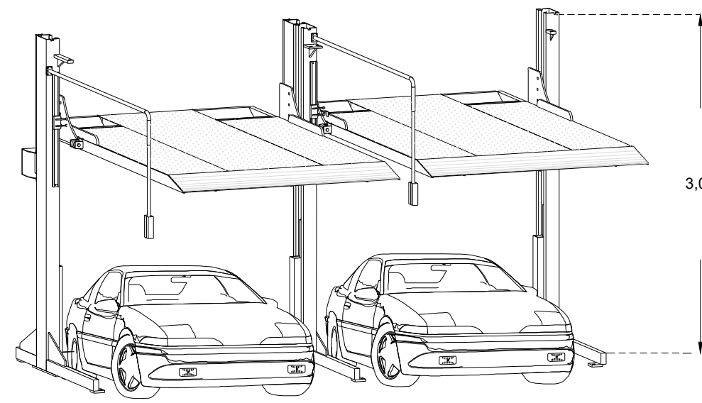
VISTA ISOMETRICO
