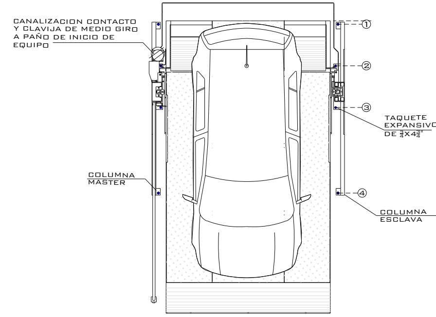
VISTA SUPERIOR
