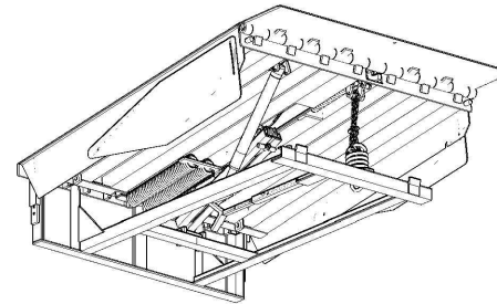
VISTA ISOMETRICO
