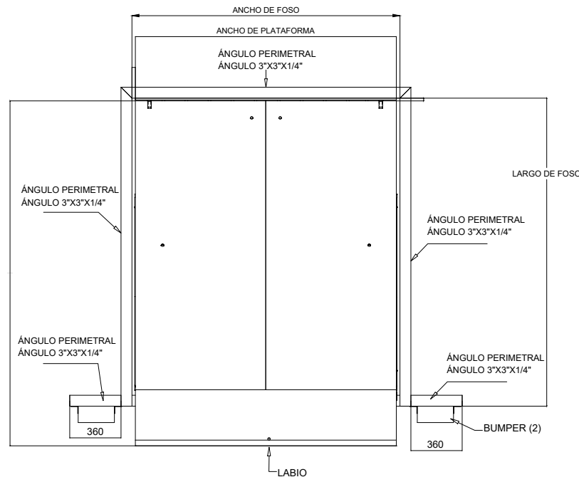
VISTA SUPERIOR DETALLE
