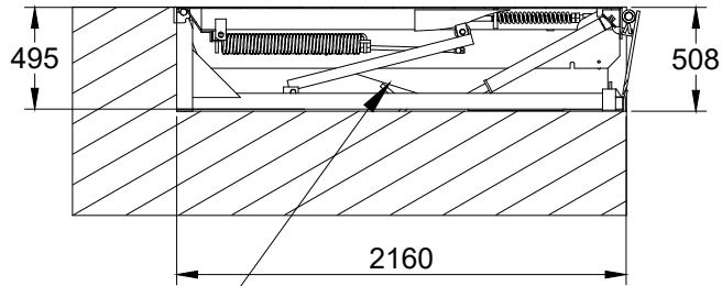
VISTA LATERAL
